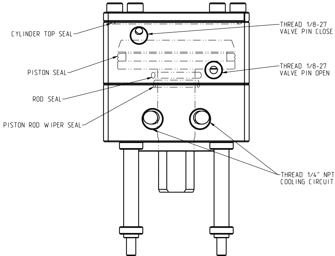
VPAC0001-A SHOWN
